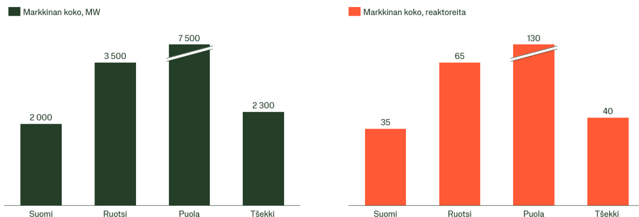
SMR-lämmön markkinapotentiaali
